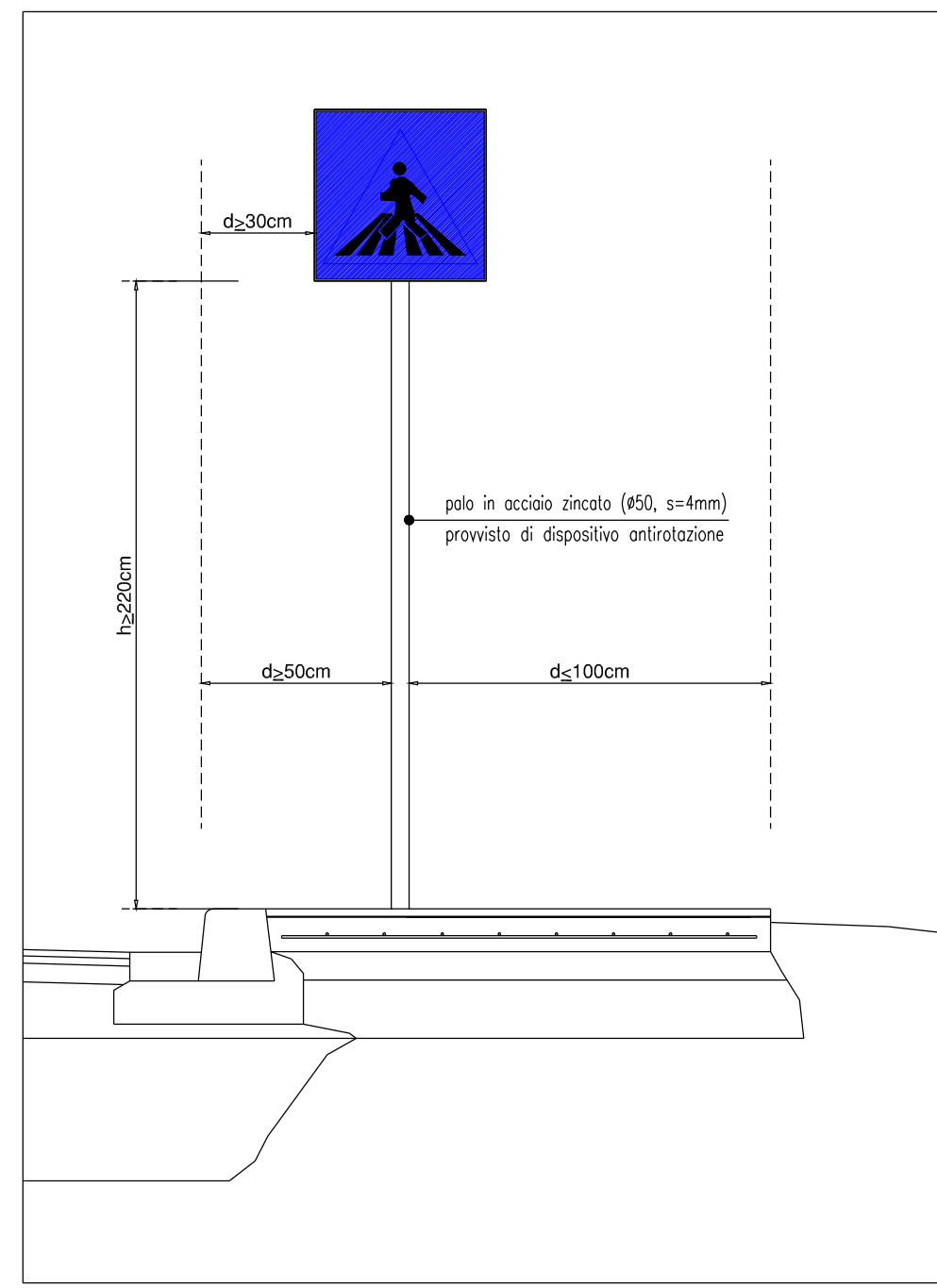
SCHEMA MONTAGGIO SEGNALETICA VERTICALE
