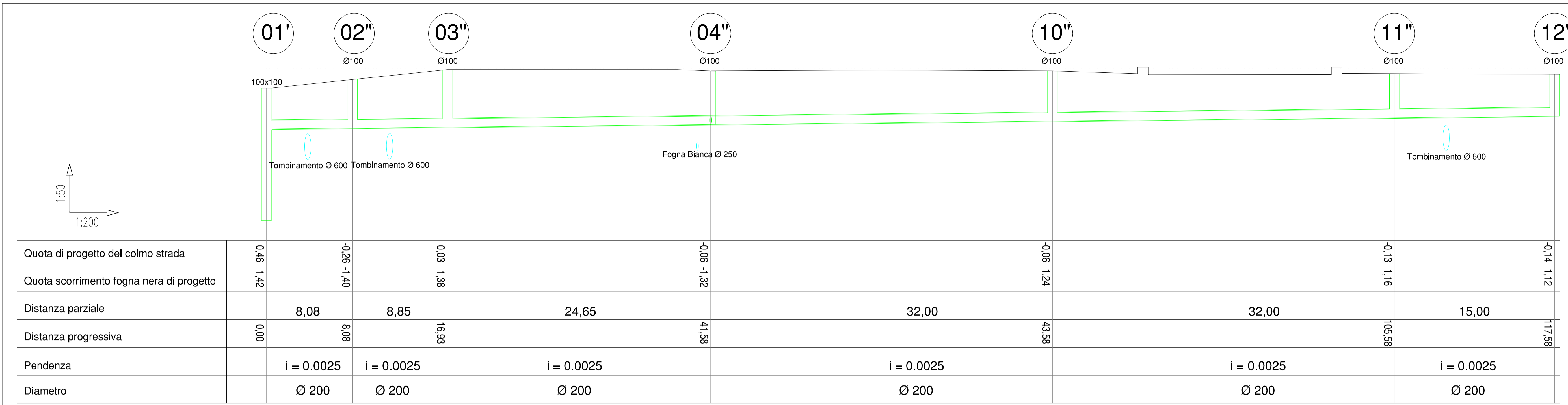
PROFILO FOGNA NERA Tratto 01''-02''-03''-04''
